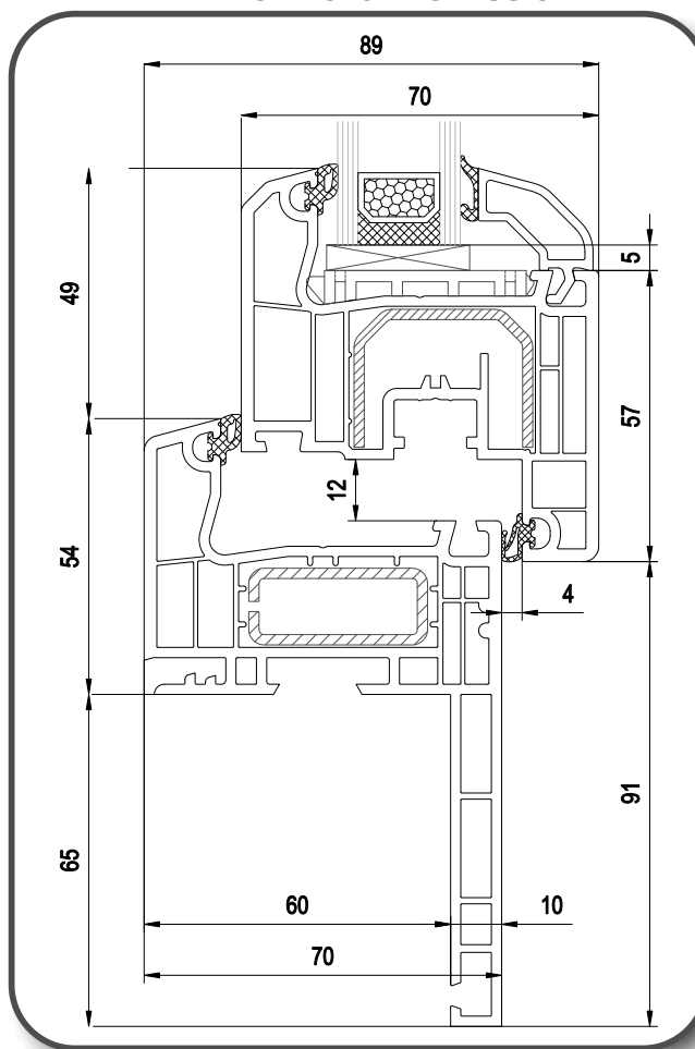
IDEAL RENOWACYJNY CLASSIC LINE
