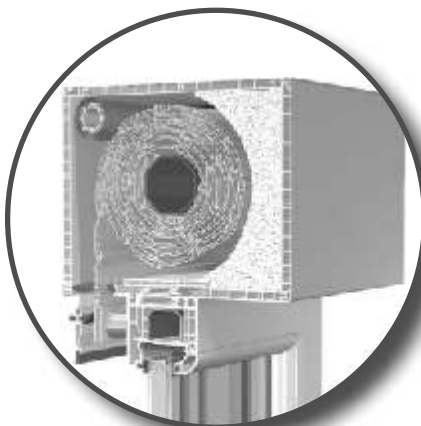
RNS ROLETY NAKŁADANE STANDARD
