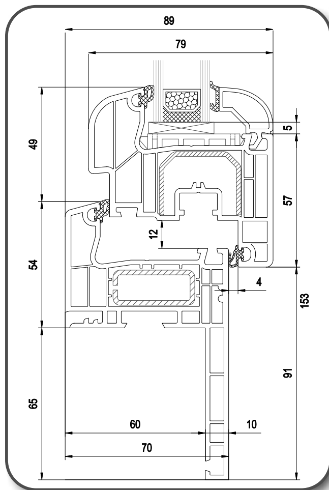
IDEAL RENOWACYJNY ROUND-LINE
